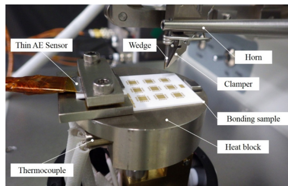
マニュアルウェッジワイヤボンダ：ワークへの実装
