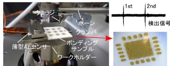
薄型AEセンサーを利用したワイヤボンディング特性評価の様子
